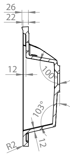
PRZEKRÓJ G-G SKALA 1 : 9
