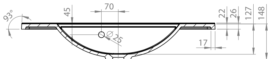
PRZEKRÓJ H-H SKALA 1 : 9
